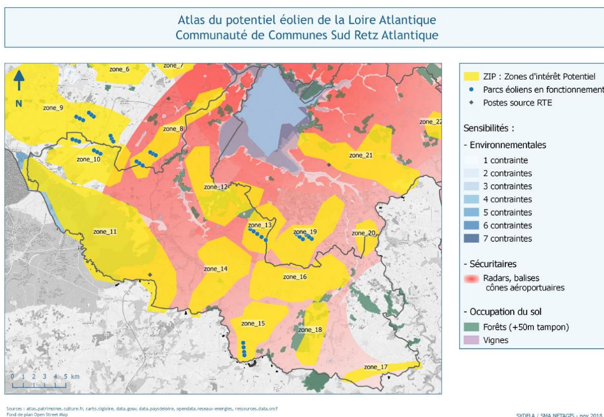
Figure 65 : Zones d'intérêt potentiel à l'implantation d'éoliennes sur le territoire de la CC Sud Retz Atlantique étude réalisée par le Sydela
