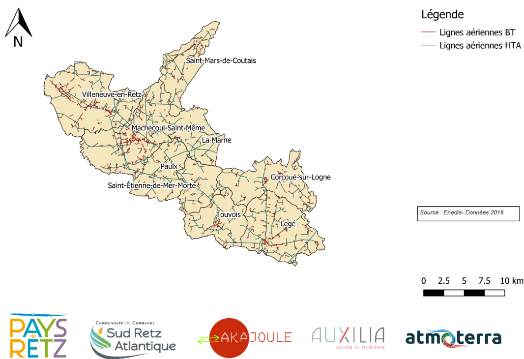
Figure 70 : Tracé du réseau de distribution d'électricité
