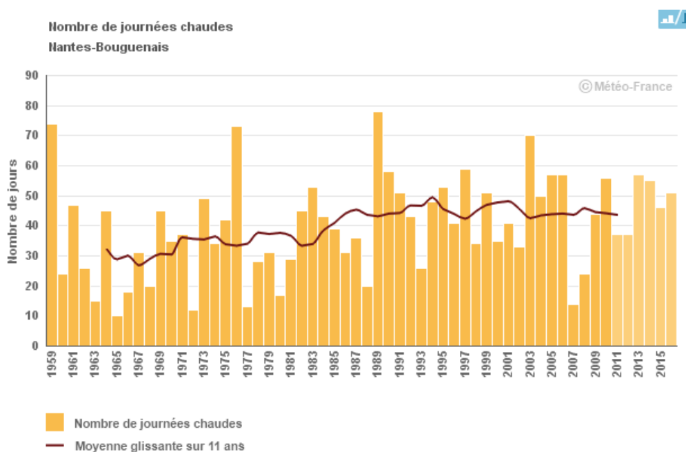
Figure 101 : Nombre de journées chaudes à Nantes-Bouguenais entre 1959 et 2016
