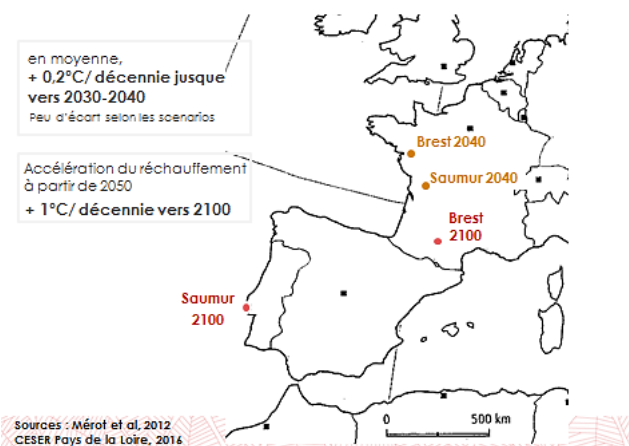
Figure 108 : Evolution des températures moyennes annuelles
