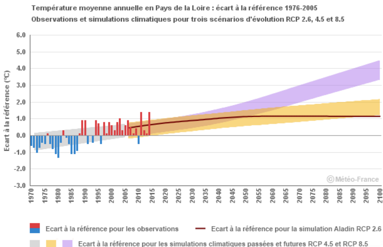
Figure 103 : Température moyenne annuelle en Pays-de-la-Loire : écart à la référence 1976-2005
