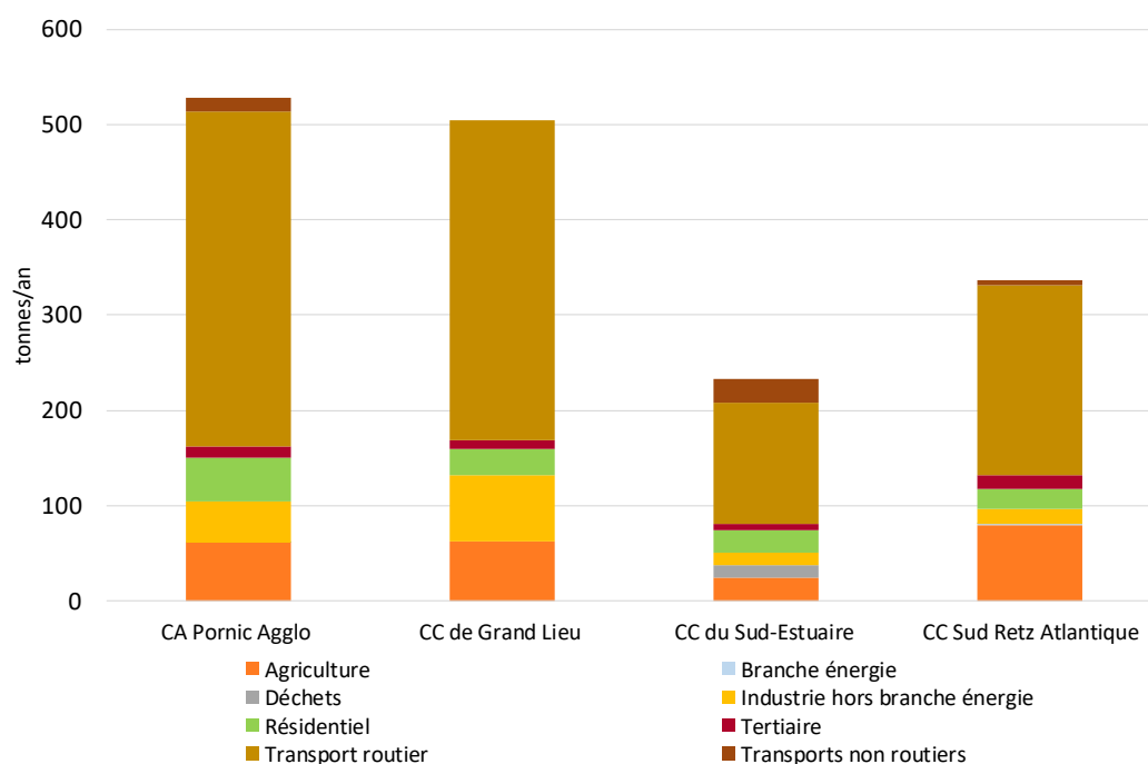
Figure 81 : Comparaison des répartitions des émissions de NO x par secteur et par EPCI en 2016
