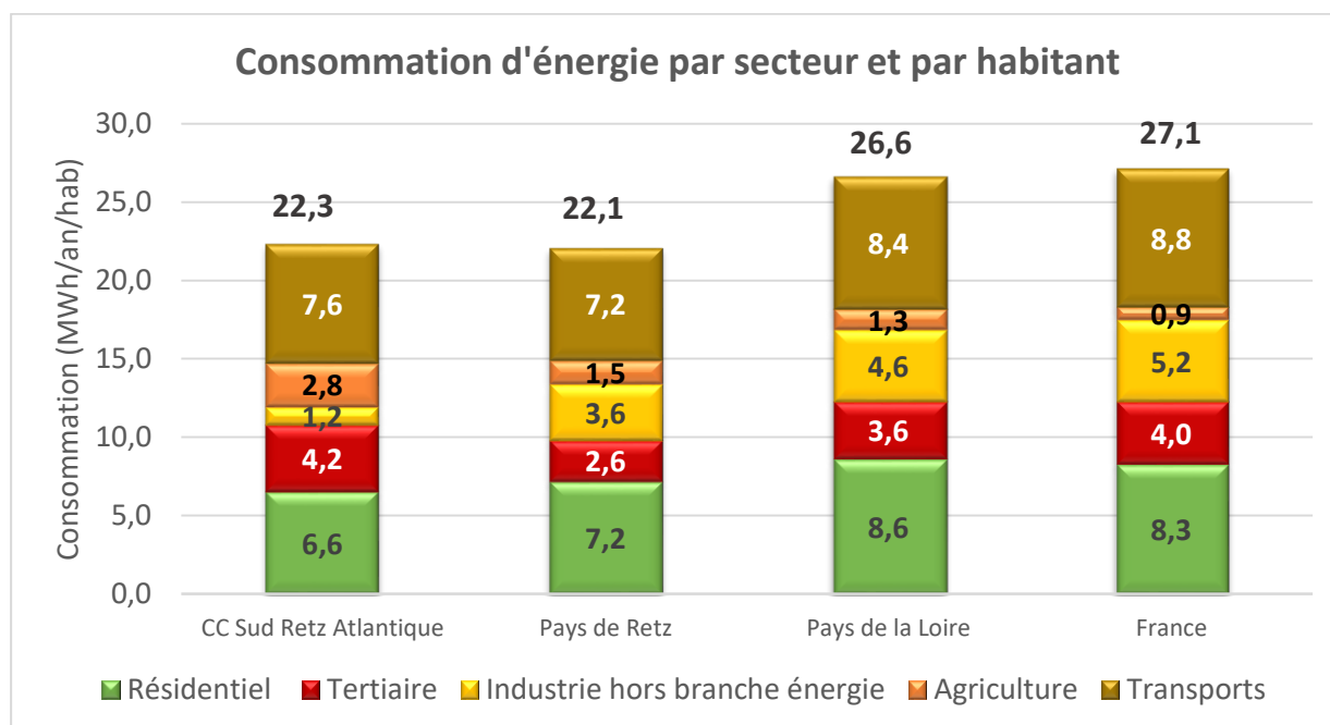
Figure 46 : Consommation d'énergie par habitant et par secteur Source : BASEMIS/Air Pays de la Loire ; SRCAE Pays de la Loire
