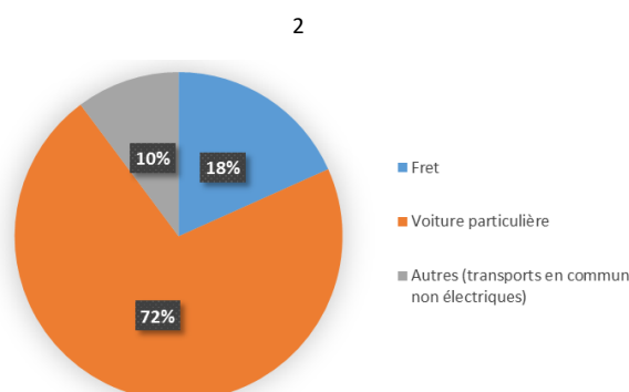
Figure 27 : Répartition des émissions énergétiques de GES du secteur routier par type de transport (à l'échelle de la CCSRA en 2016)
