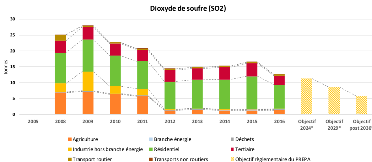
Figure 86 : Evolution des émissions de SO 2
