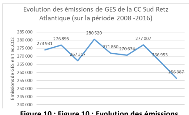
Figure 10 : Evolution des émissions territoriales de GES de la CCSRA sur la période 2008-2016
