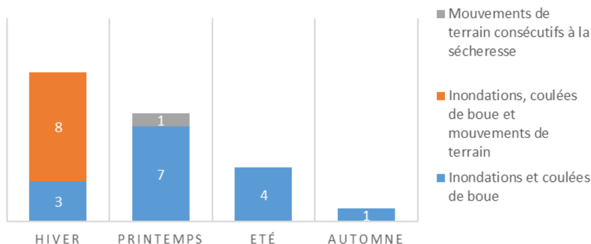
Figure 112 : Arrêtés de catastrophes naturelles sur le territoire de la CCSRA entre 1983 et 2016 Source : Outil Impact Climat sur la base des données GASPAR
