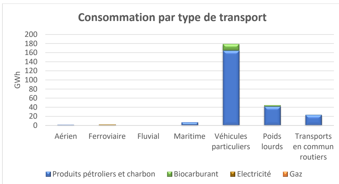
Figure 54 : Consommation énergétique par type de transport et d'énergie
