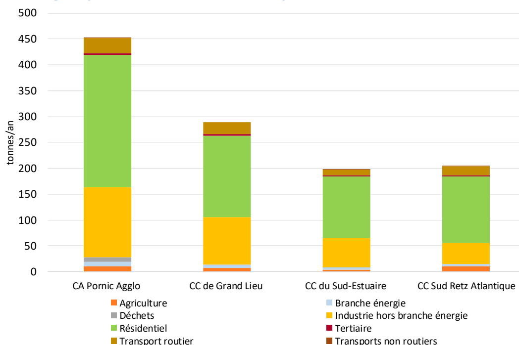
Figure 84 : Comparaison des répartitions des émissions de COVNM par secteur et par EPCI en 2016
