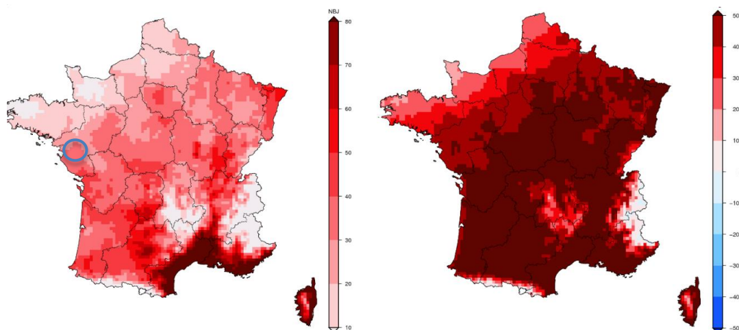
Figure 106 : Nombre de nuits tropicales pour le scénario 8.5, horizon 2071-2100, moyenne annuelle
