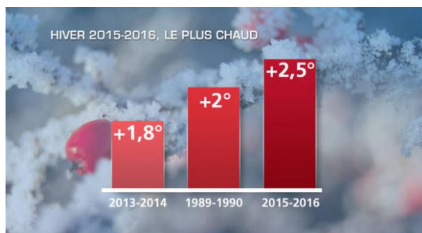
Figure 11 : Ecart par rapport à la température moyennée de référence (1981-2010)
