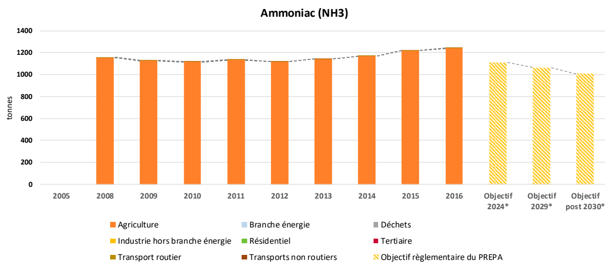
Figure 90 : Evolution des émissions de NH 3 Source : BASEMIS / AIR PAYS DE LA LOIRE
